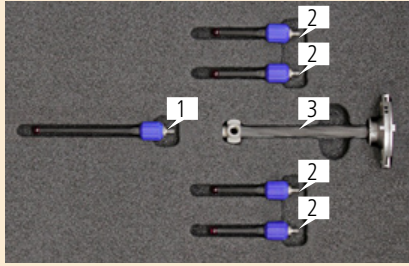
带滚花测针的星形测针组合 TL3 型号: 626103-9043-000
