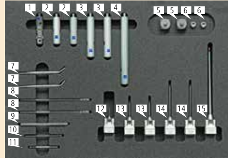
标准测针套件, M5 型号: 626115-9100-000 1
