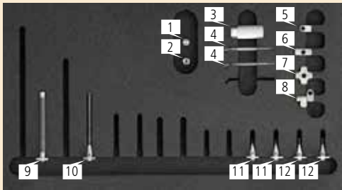
测针组合4 VAST XXT, 小 型号: 626103-9024-000
