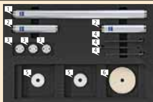
盘形测针套件 型号: 626115-9160-000
