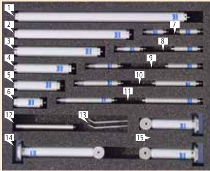
ThermoFit 测针和加长杆套件 型号: 626107-9010-000
