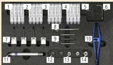
星形测针套件, M5 型号: 626115-9140-000
