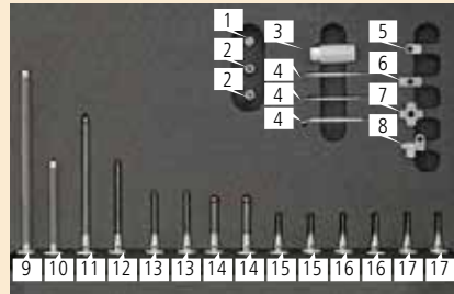
测针组合5 VAST XXT, 大 型号: 626103-9025-000
