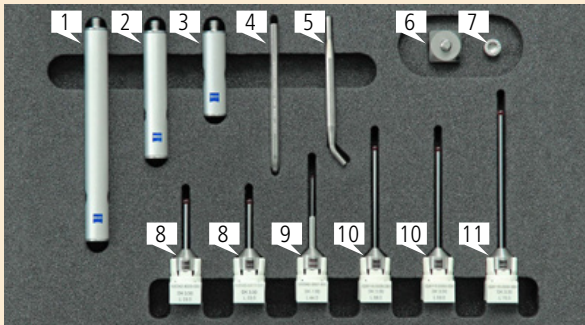
基本测针套件, M5 型号: 626115-9170-000
