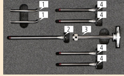
测针保持架组合 TL3, 长 型号: 626103-9058-000
