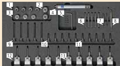
小型星形测针套件, M5 型号: 626115-9150-000
