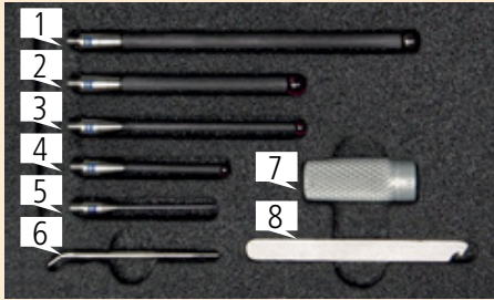
测针组合1 VAST XXT, 适用于小工件 型号: 626103-9021-000
